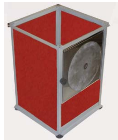
30 701 05 Tisch für Profi-Beveler mit Aufbe- wahrungskassette für 8 Magnet- scheiben Table for Profi-Beveler with Storage- case for 8 magnetic discs
